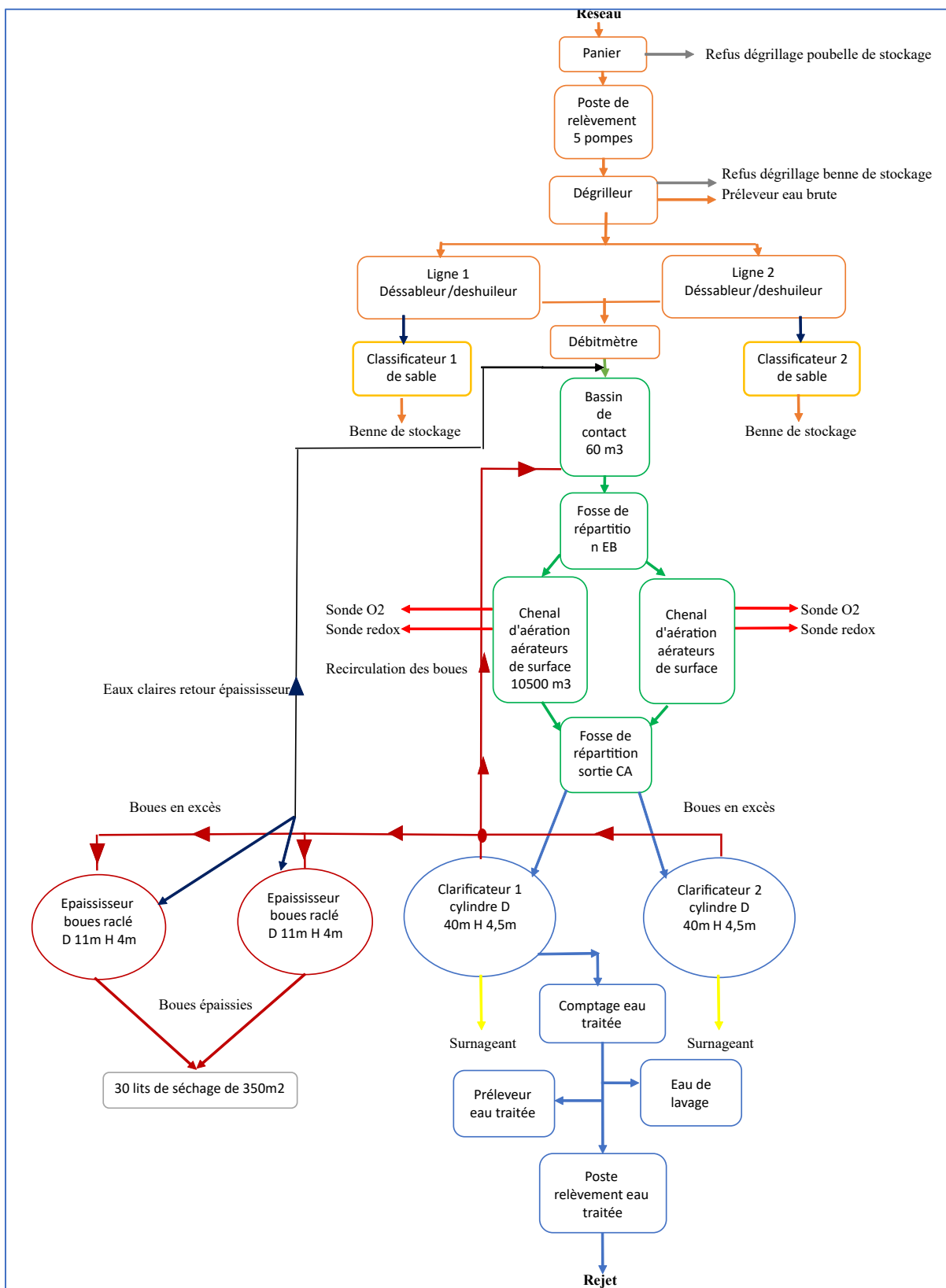
Figure 10 : Synoptique de fonctionnement de la STEP de Sfax Nord
