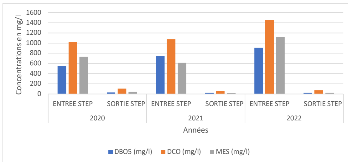
Figure 28 : Concentrations annuelles moyennes : DBO5, DCO et MES (SEGOR : Rapports mensuels d'exploitation de la STEP Sfax Nord)
