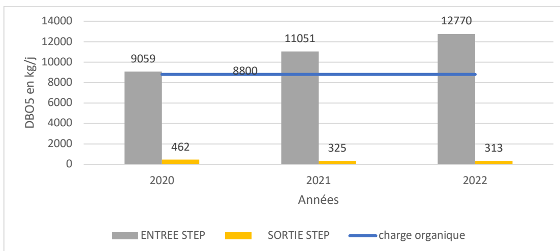
Figure 29 : Taux de saturation organique de la STEP de Sfax Nord (SEGOR : Rapports mensuels d'exploitation de la STEP Sfax Nord)
