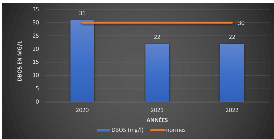
Figure 30 : Concentrations annuelles moyennes en DBO5 des eaux épurées de la STEP de Sfax Nord (SEGOR : Rapports mensuels d'exploitation de la STEP Sfax Nord)
