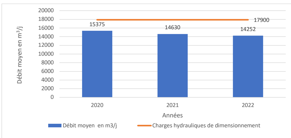
Figure 27 : Saturation hydraulique de la STEP de Sfax Nord (SEGOR : Rapports mensuels d'exploitation de la STEP Sfax Nord)
