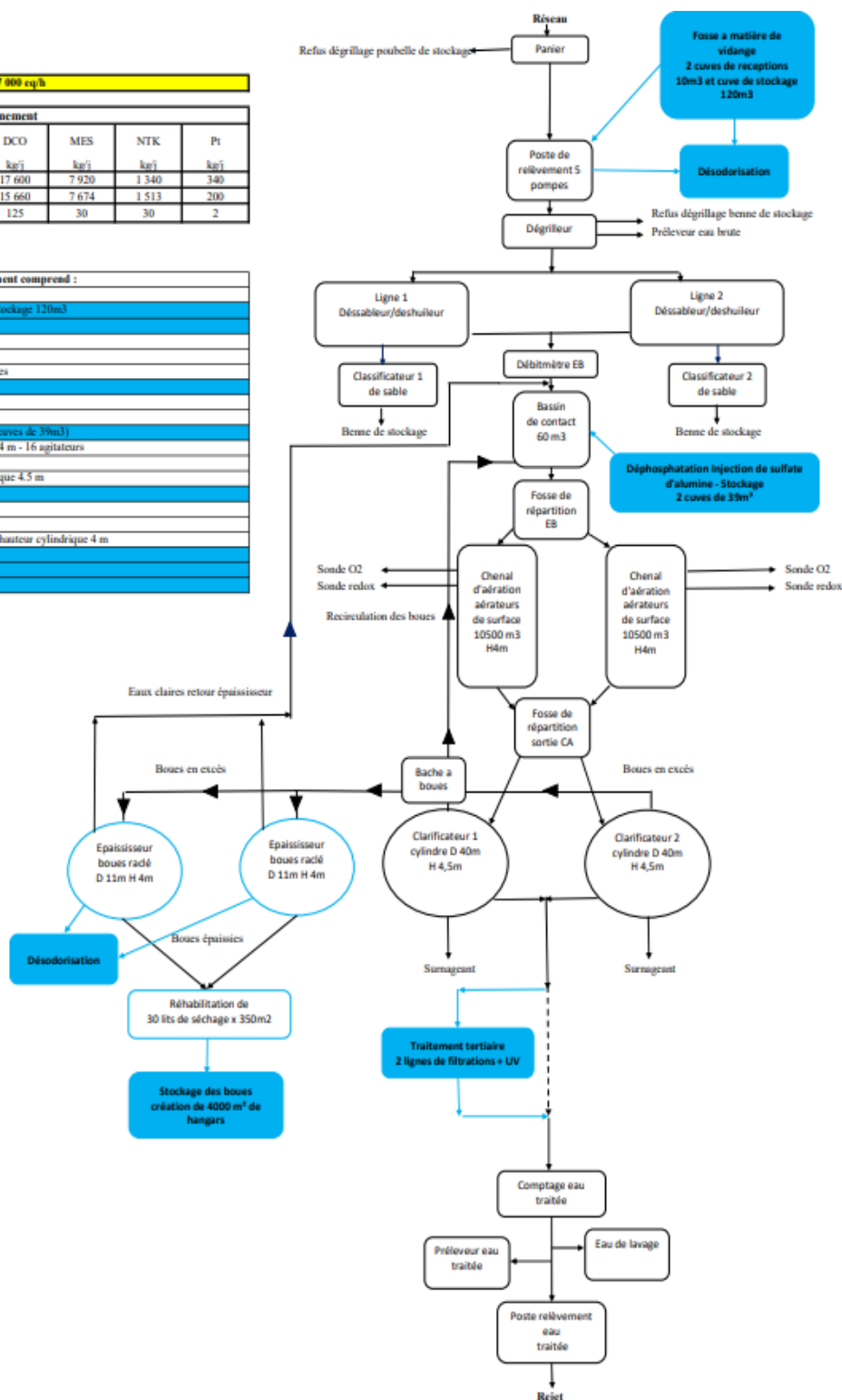
Figure 42 : Schéma global de fonctionnement la STEP de Sfax Nord suite aux aménagements projetés
