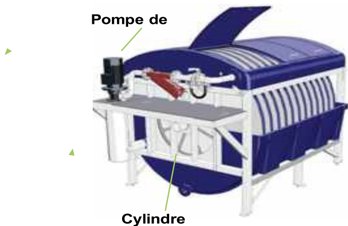
Figure 37 Schéma d'un CompakblueTM avec un capot ouvert montrant le haut des disques
