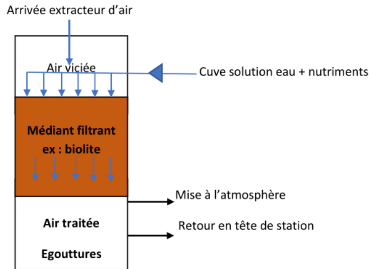
Figure 41 : Schéma de principe de traitement d'odeur
