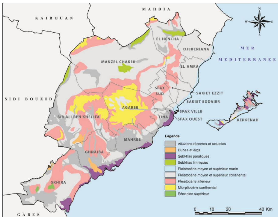
Figure 49: Carte géologique de Sfax (Atlas du gouvernorat de Sfax, 2013)
