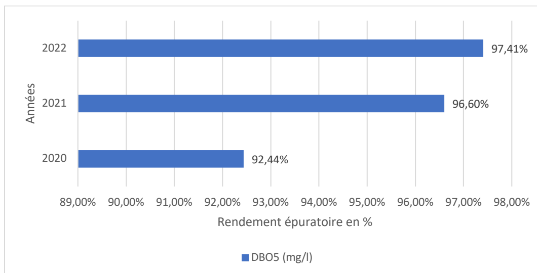
Figure 31 : Rendement épuratoire en DBO5 (SEGOR : Rapports mensuels d'exploitation de la STEP Sfax Nord)
