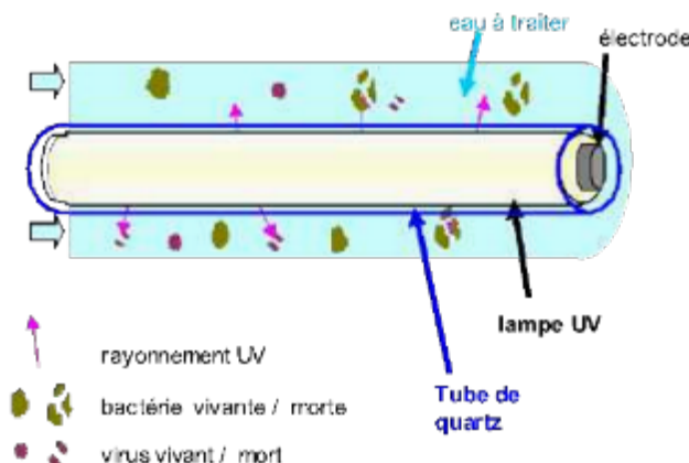
Figure 39 : Schéma de fonctionnement des lampes UV
