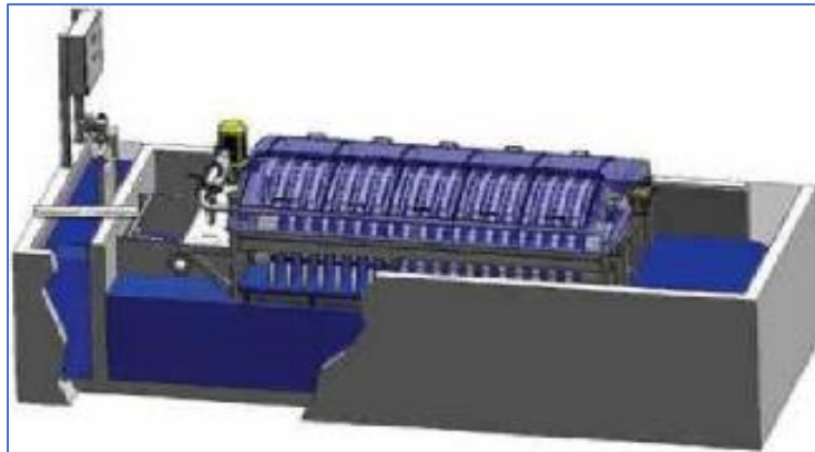
Figure 36 - Exemple d'appareil à installer en cuve béton
