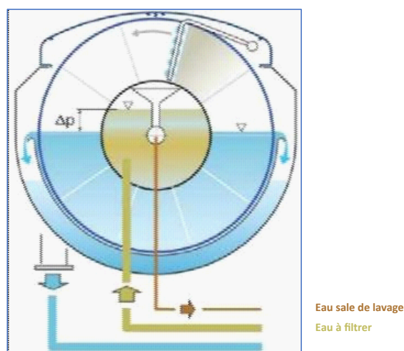
Figure 38 - Circuit des différentes eaux (propre et sale)
